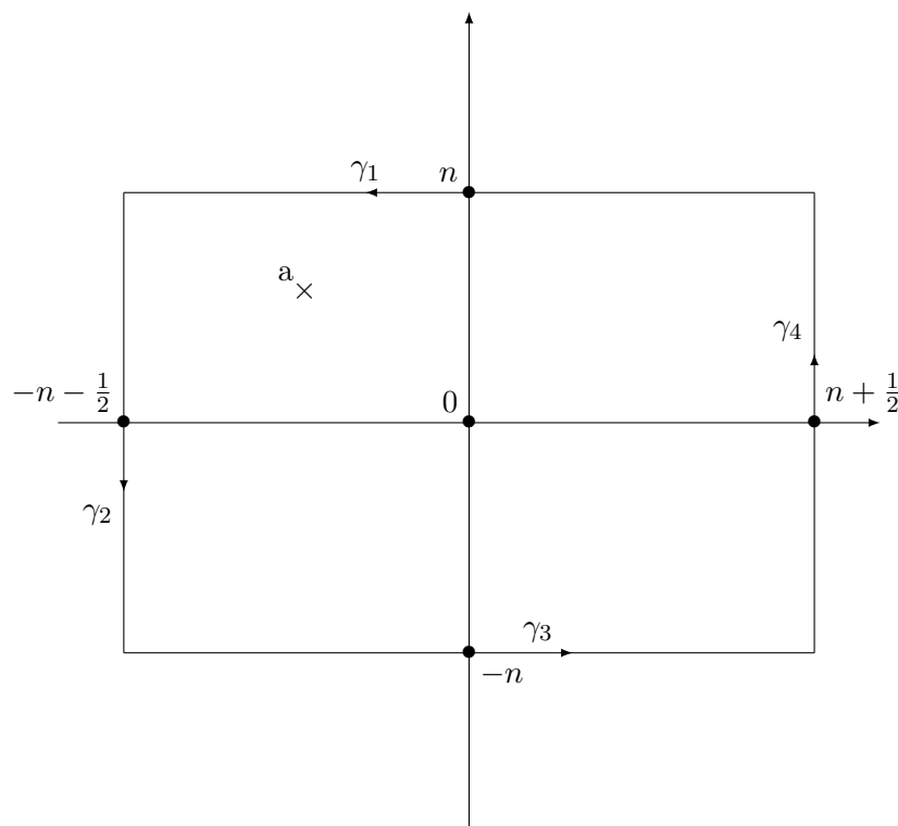
FIGURE 1 – Contour d'intégration pour la formule de la cotangente
